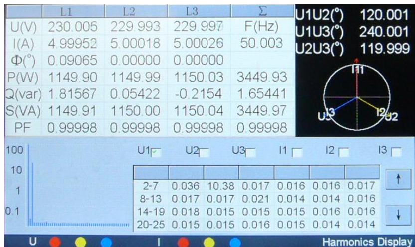
图 11 谐波显示
